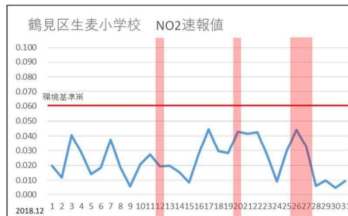
子安台換気所 NO2除去率が低下した日
