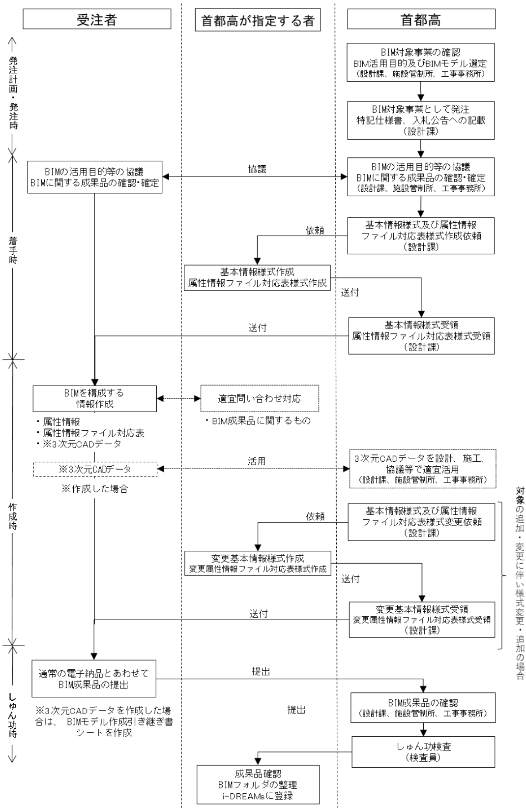
図-6 BIM 対象事業における発注～しゅん功までの作業フロー
