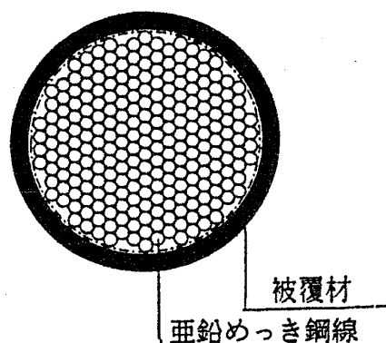
図 3.2.10-1 断面の概要
