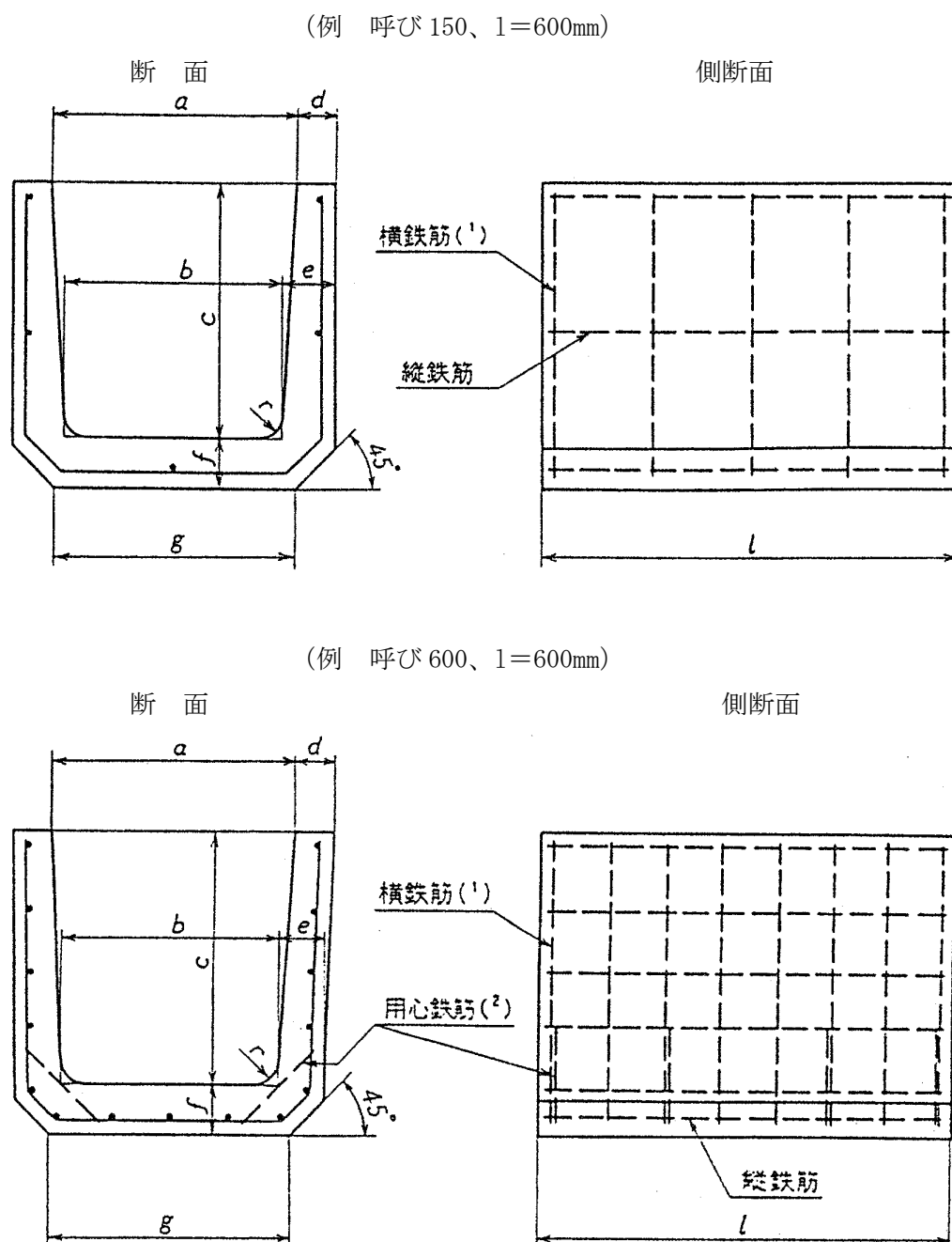
図 4.2.6-1 本体の形状、寸法及び配筋
