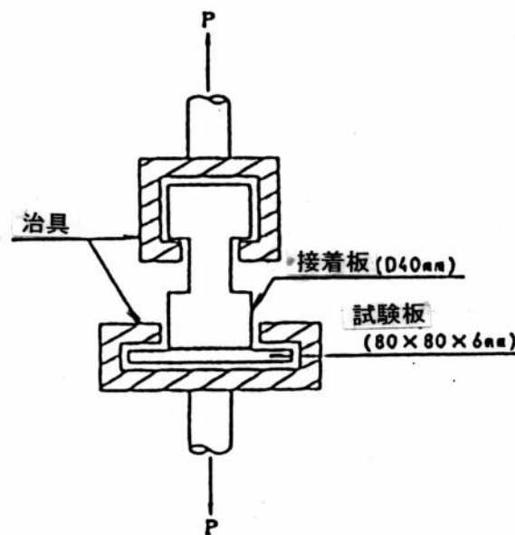
図 6.15-3 接着力試験
