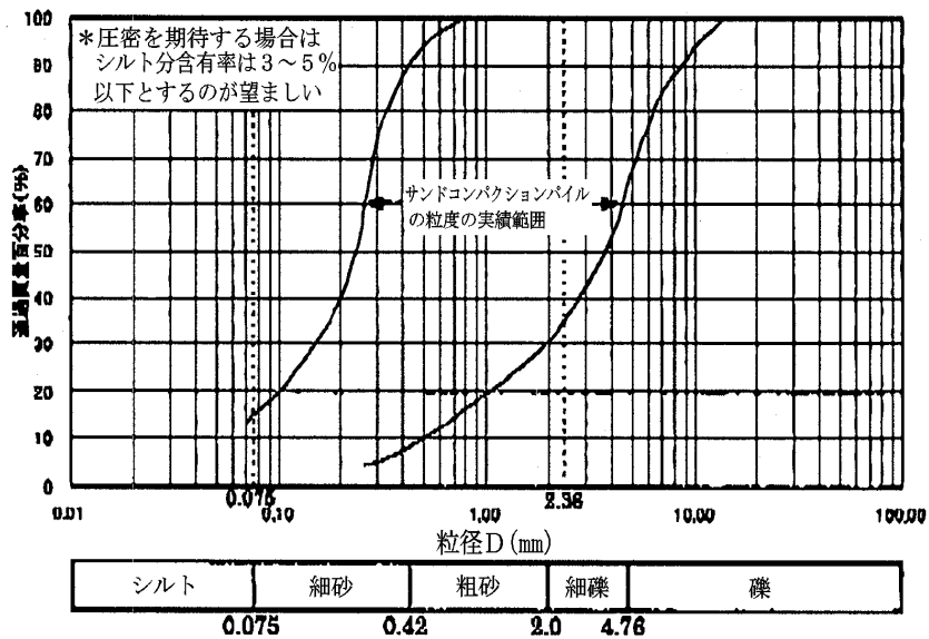
図 3.2 S C P 砂杭材料の粒度実績範囲
