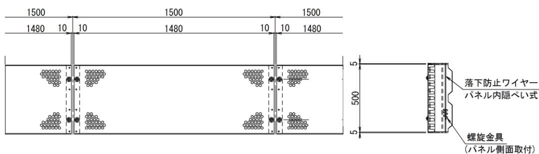
図-8.7-2 改良型吸音板
