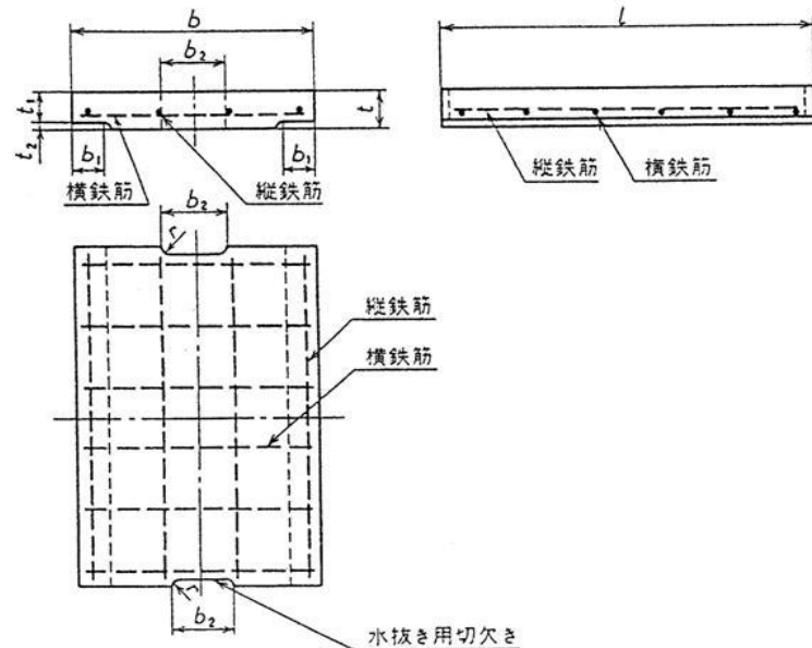
図 4.2.6-2 ふたの形状、寸法及び配筋
