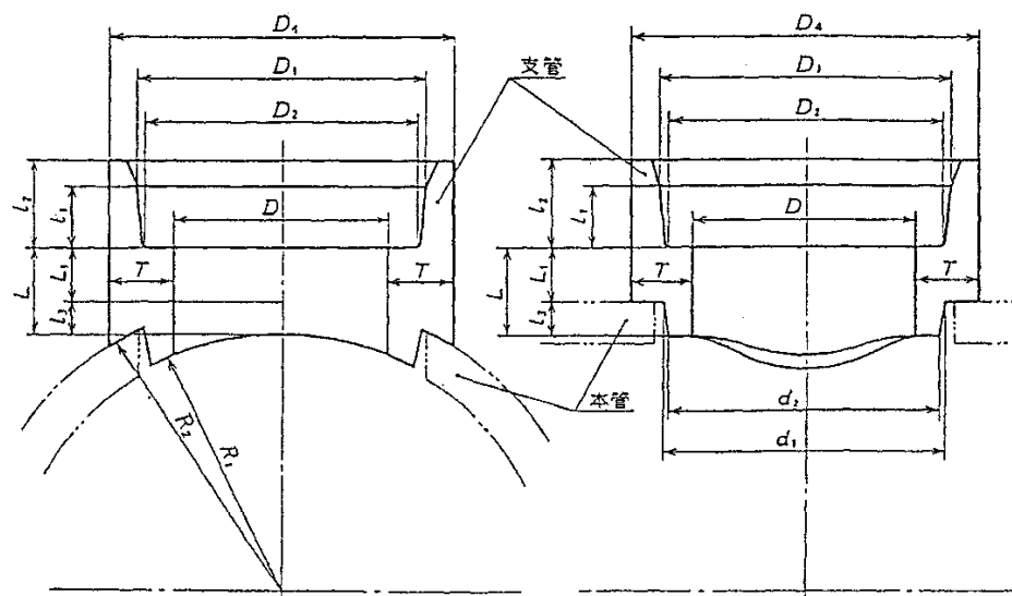
图 4.2.5-2 形状 支管
