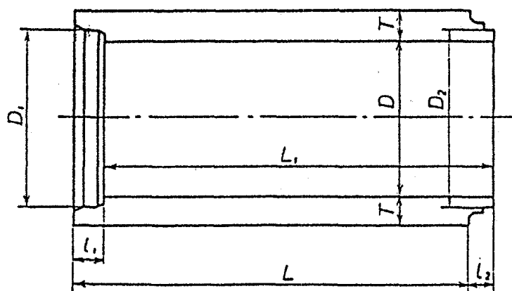
図 4.2.5-1 形状 NC形
