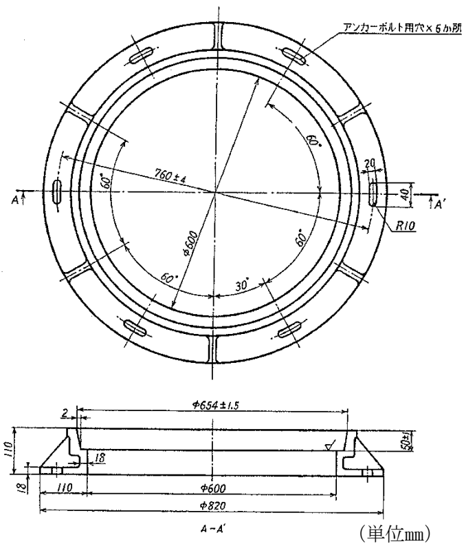
図 4.2.7-4 球状黒鉛鑄鉄の枠 (平受けφ600mm用)
