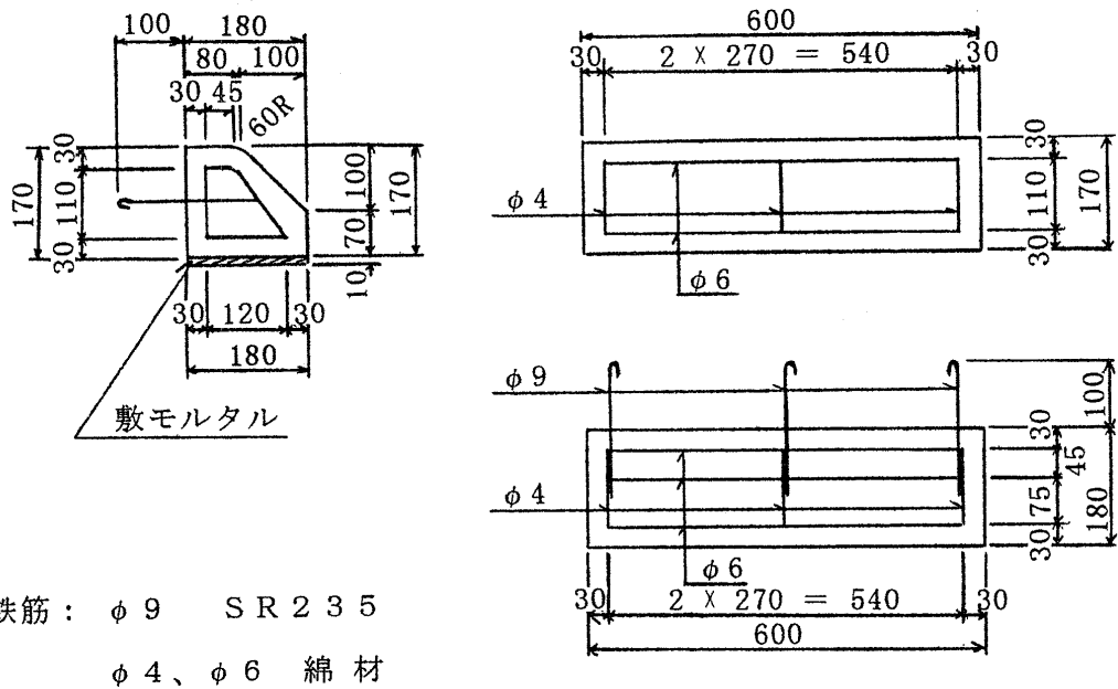
図 4.2.8-1 形状、寸法及び配筋
