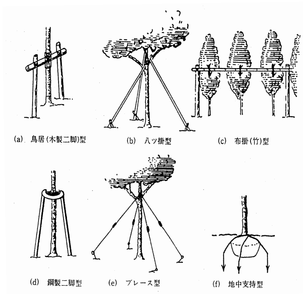
図 7.5-1 支柱形式
