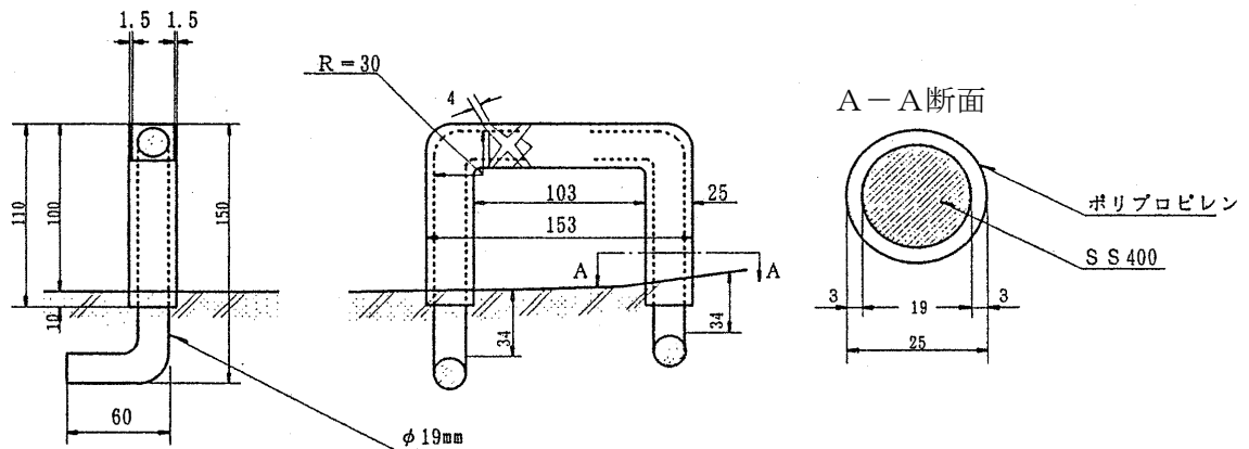
図 4.2.7-2 足掛け金物の形状、寸法
