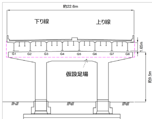
図-3 断面図（小-307～小-308橋脚）
