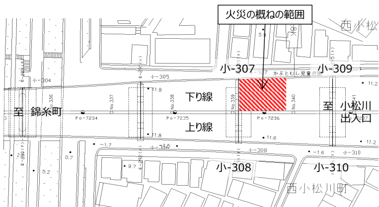
図-2 平面図
