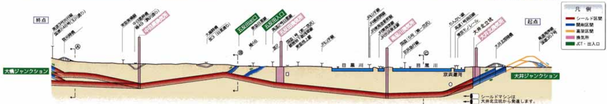
① シールドトンネル 出入口 概略図 (概略図)
