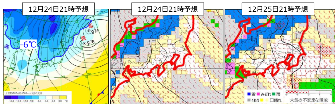
地上天気図 上空約1500m付近の気温 青実線：-6℃は平地で雪となる目安
