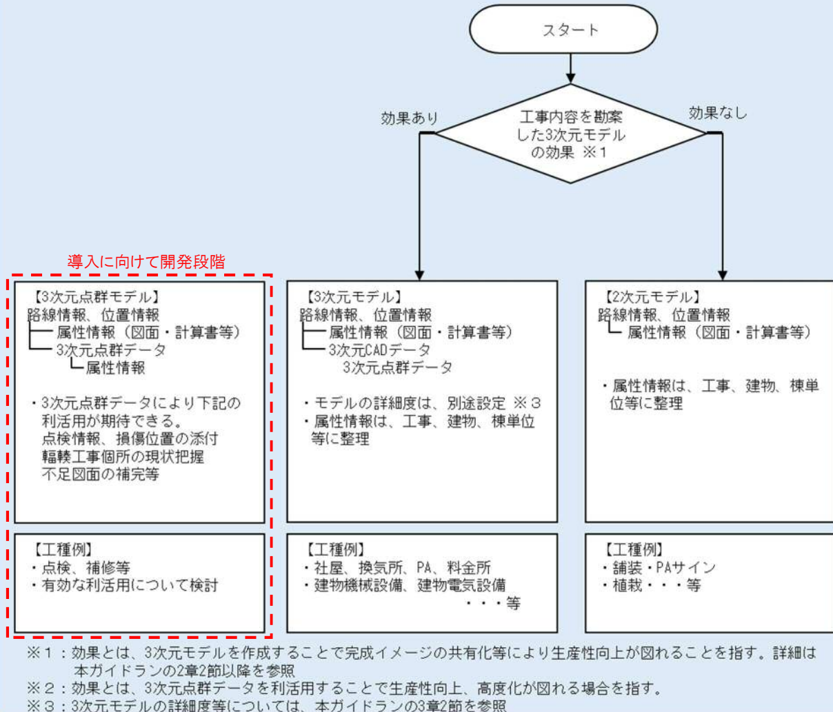
図3. BIM/CIMモデル選定の基本フロー
