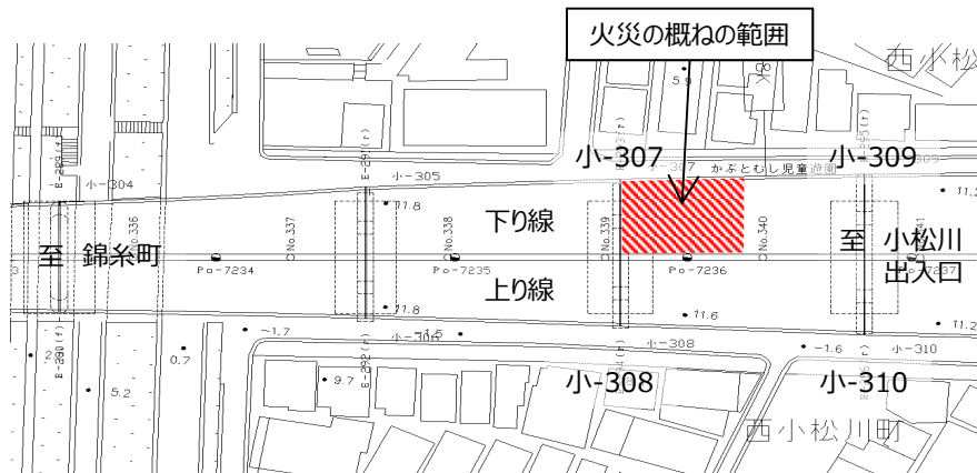
平面図
