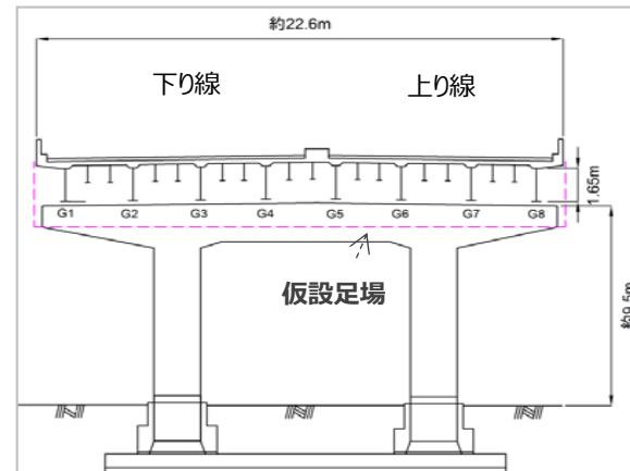
断面図（小-307～小-308橋脚）
