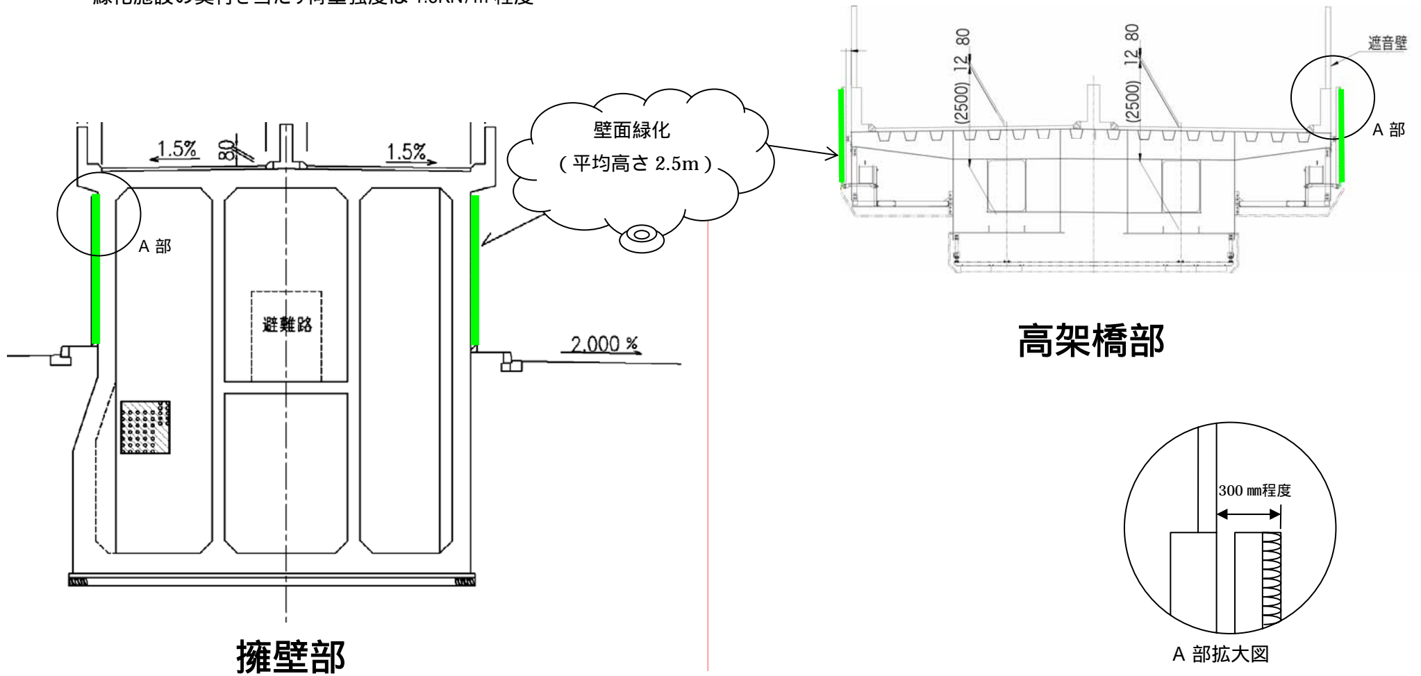
別紙 - 2 壁面緑化概要図
