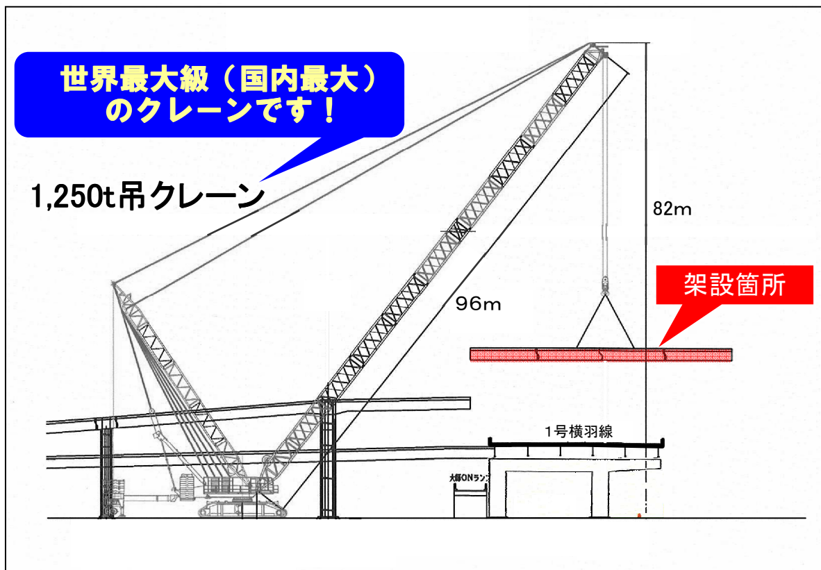
《架設状況図》
