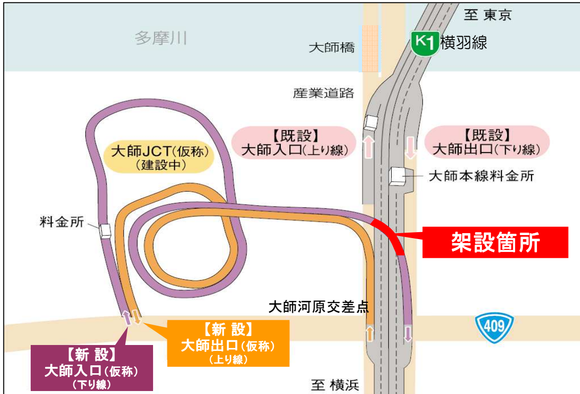
《架設箇所図》
